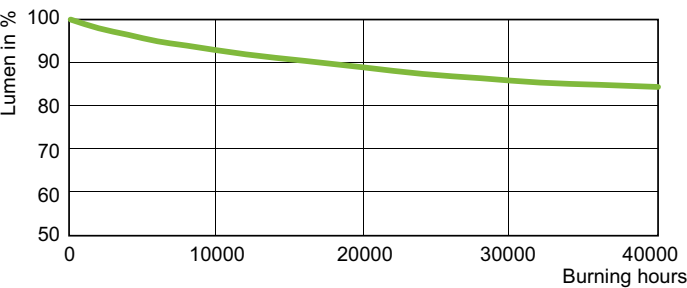
Lumen Maintenance Diagram - MST SON APIA Plus Xtra 100W E40 1SL/12
