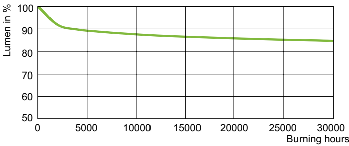
Lumen Maintenance Diagram - MASTER SON PIA Plus 70W/220 I E27 1CT/24
