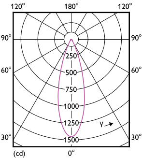
LEDspots MAS IC 6,7W MR16 GU5,3 930 36D-LDD
