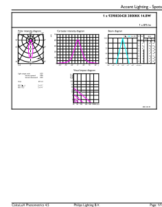
LEDspots MAS SLR 14,8W AR111 G53 930 24D-ADL ADL
