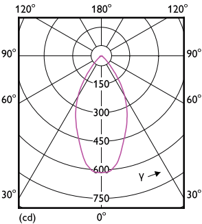
LEDspots MAS IC 6,7W MR16 GU5,3 930 60D-LDD
