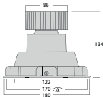
Rund - Mono HO
