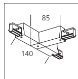
T - Verbinder
