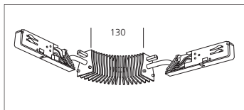
Flexibler Verbinder
