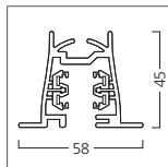
Einbau-Schieneneneinheit
