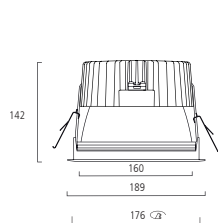
Abmessungen (mm)
