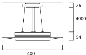
Abmessungen
