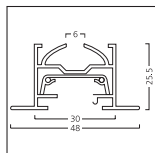
Einbau-Schiene
