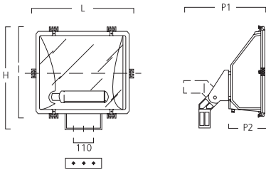
Betriebsgeräteeinsetz HSI-T 1000/2000 oder SHP-T 1000
