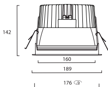
Abmessungen (mm)
