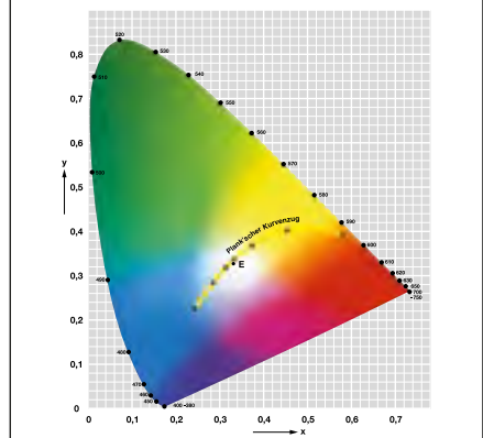
Normfarbtafel nach DIN 5033
