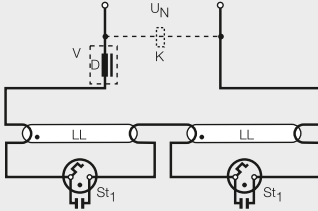
Bild 2 Reihenschaltung für zwei Lampen 4 W, 6 W, 8 W, 15 W, 18 W, 20 W und 22 W an 220 V – nur mit Starter ST 151 + ST 172 (s. Seite 6.38)
