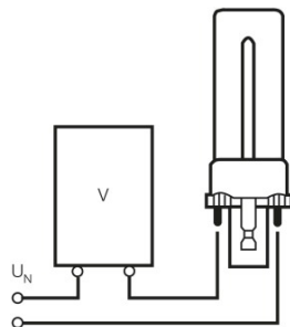
Schaltplan
